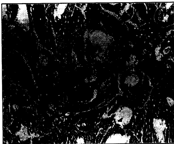
تصویر ۶- نمونه کالوس از حیوانات گروه آزمایش در روز ۹۰ (رنگ آمیزی H&E، x۱۲۳). (a) تیغه های استخوانی، (b) سیستمهای هاورس.
