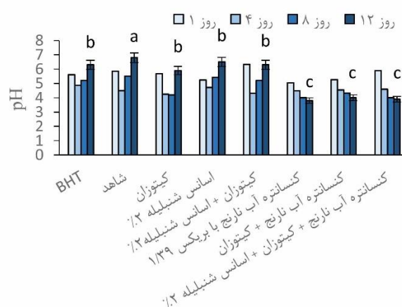
تصویر ۳. تغییرات PH نمونه‌های مختلف در مدت زمان نگهداری ۱۲ روز در دمای یخچال.
