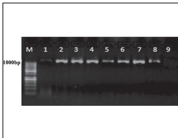
تصویر ۲. ژل آگارز ۲٪ مربوط به PCR حاصل از قطعه M = ۱۶S rDNA RFLP. مارکر = ۵۰ bp. ۱-۸ = ایزوله‌های مورد آزمایش، ۹ = کنترل منفی (لاکتو کوس گارویه (Accession No: X۵۴۲۶۲).
