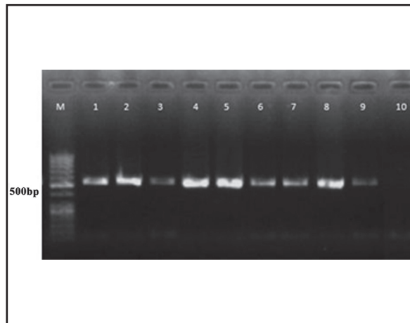
تصویر ۱. ژل آگارز ۲٪ مربوط به PCR حاصل از DNA برخی ایزوله‌های استرپتو کوس اینیایی بدست آمده در تحقیق. M = مارکر = ۵۰ bp. ۱-۸ = ایزوله‌های مورد آزمایش، ۹ = کنترل مثبت (استرپتو کوس اینیایی: Accession No AF۰۴۸۷۷۳). ۱۰ = کنترل منفی (لاکتو کوس گارویه X۵۴۲۶۲). (Accession No: X۵۴۲۶۲).
